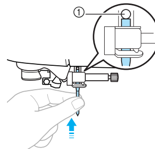
① Nadelanschlag
