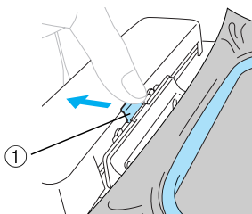
① Zum Abnehmen hier drücken.
