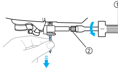
① Schraubendreher ② Nadelklemmschraube
