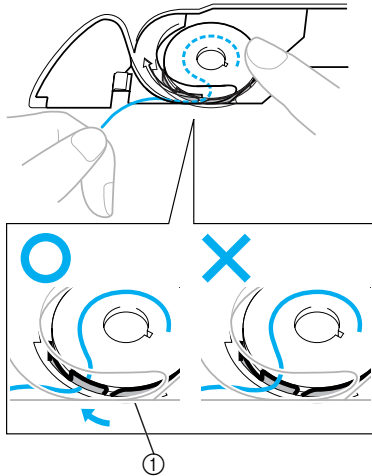
① Spannungseinstellfeder
