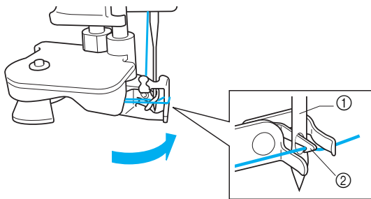
① Nadel ② Haken
