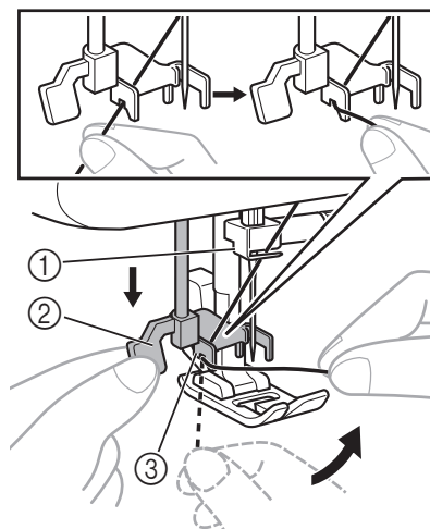
① Nadelhalter ② Nadeleinfädlerhebel ③ Führung
