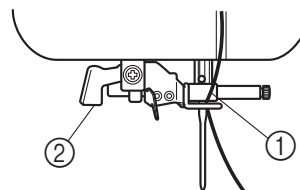
① Nadelhalter ② Nadeleinfädlerhebel
